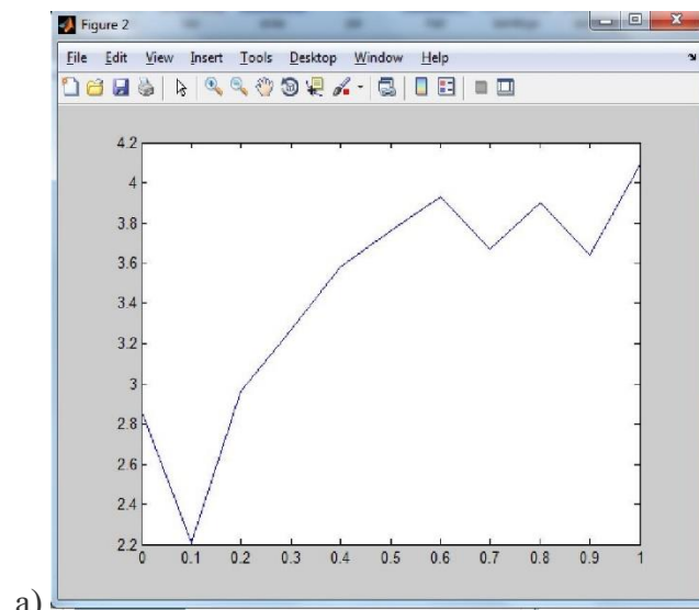
a) Рисунок 1 – график исходной функции
