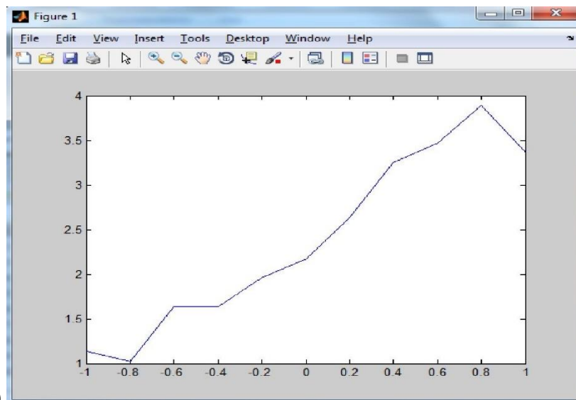
Рисунок 6 – график исходной функции
